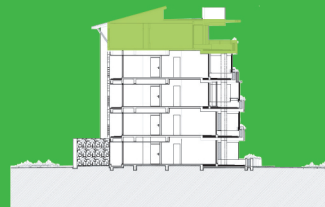
SECCIÓN ESQUEMÁTICA SCHEMATIC SECTION
